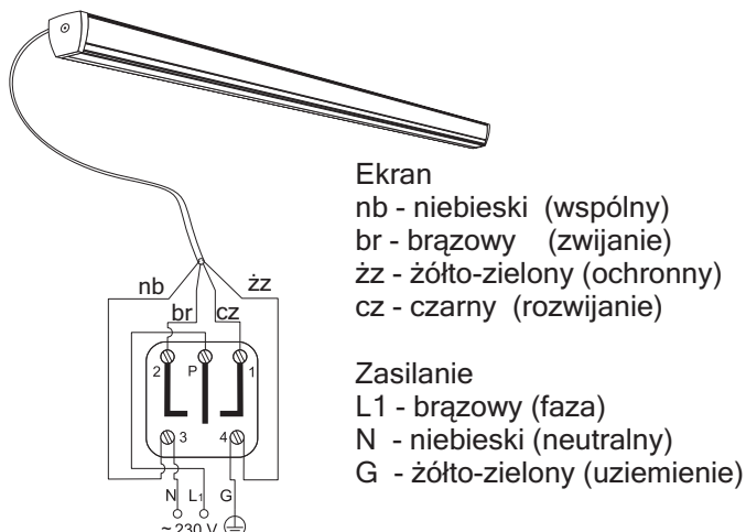
Rys.9 Schemat podłączenia ekranu (bez zdalnego sterowania)
