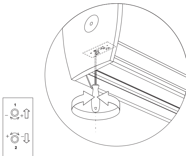
Rys.11 Regulacja położenia dolnej listwy ekranu
