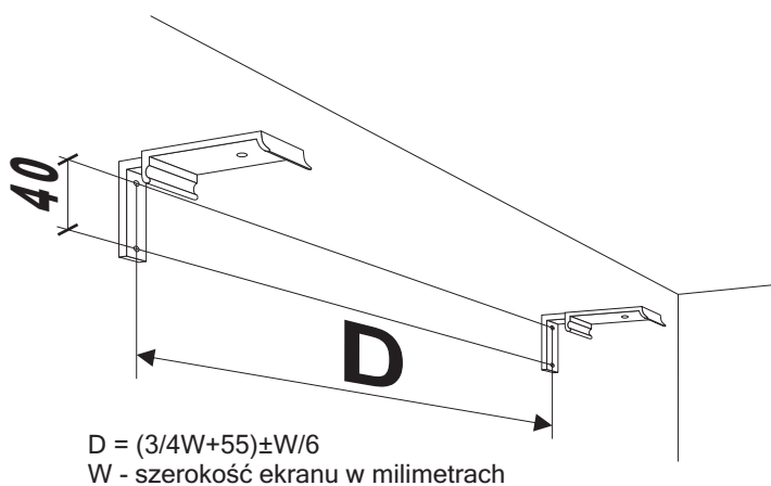
Rys.5 Mocowanie uchwyty ścienne ekranu
