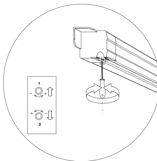
Rys.6 Regulacja ekranu
