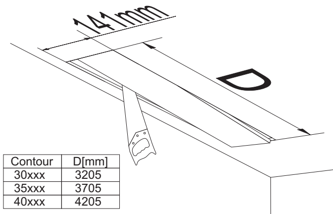
Rys.5 Przygotowanie otworu dla modułu sufitowego
