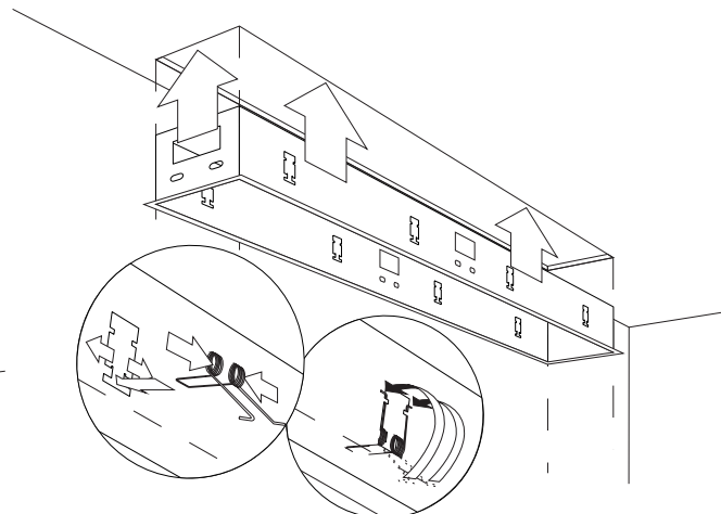
Rys.6 Montaż modułu sufitowego
