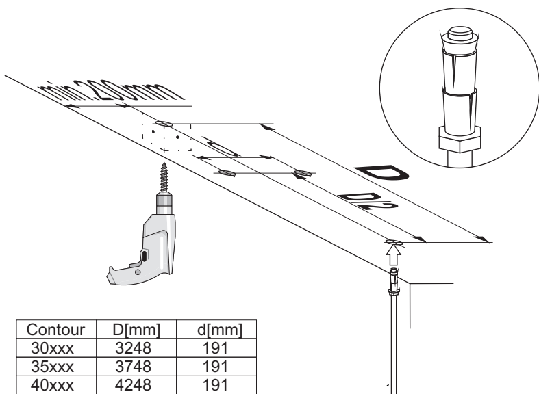
Rys.1 Instalacja szpilek mocujących w suficie
