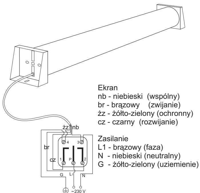
Rys.9 Podłączenie sterowania ekranu
